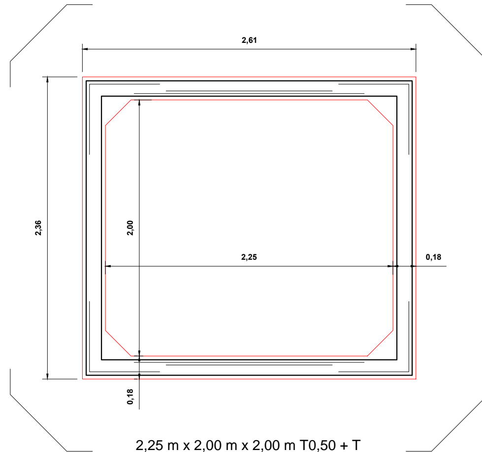
ARMADURA TRANSVERSAL Y LONGITUDINAL
